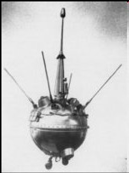
sonda Luna 2 ( 1959 )
