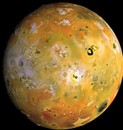
Io
