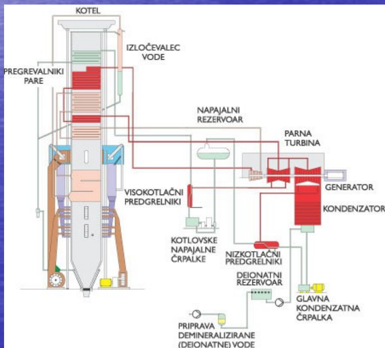
SHEMA TERMOELETRARNE
