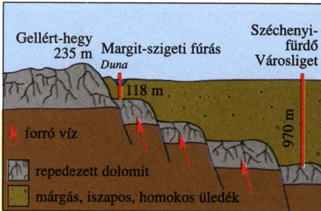
A főváros hévizzforrásainak útja
