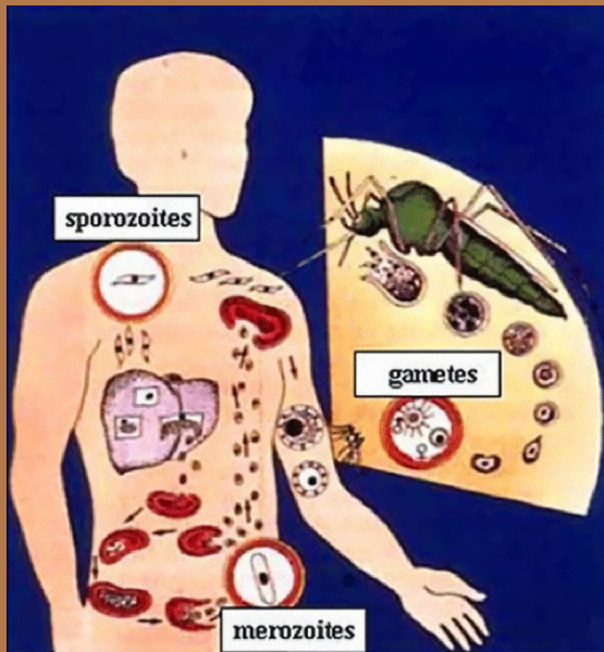
Cikel malarije
