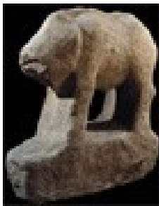
Slika 6: Granitni bik
