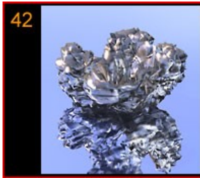
Slika 10: Molibden v elementarnem stanju
