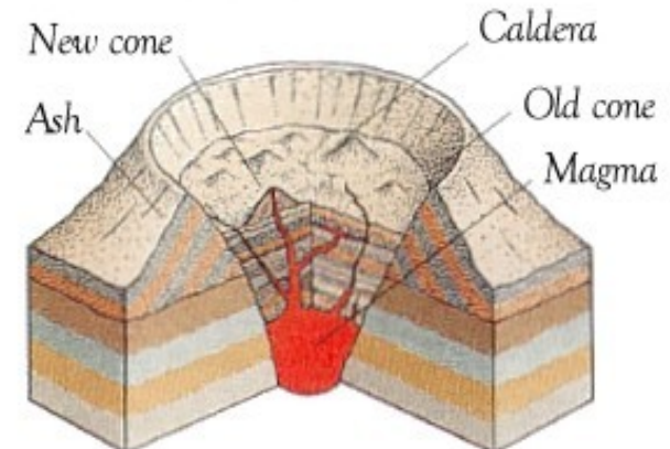
Caldera volcano
