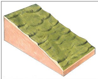
Soliflukacija
