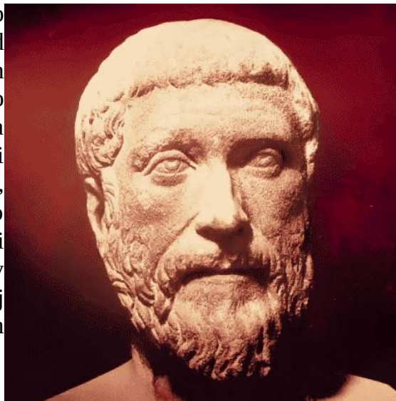
Slika 2: Pitagora
