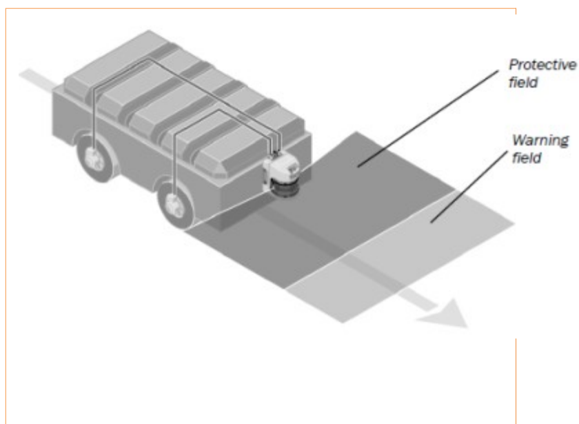
Slika 13.8: Prikaz varovanja
