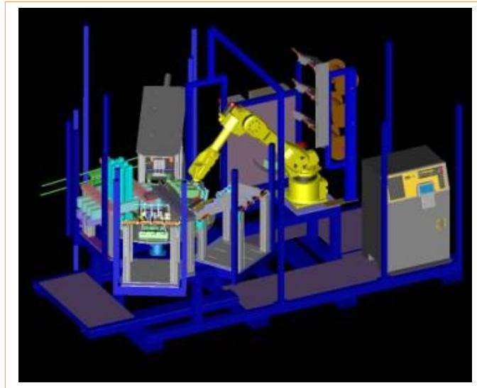
Slika 15.2: Izris robotske celice
