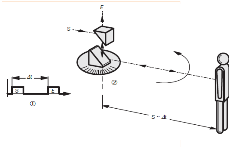
Slika 13.7: Delovanje optičnega senzorja
