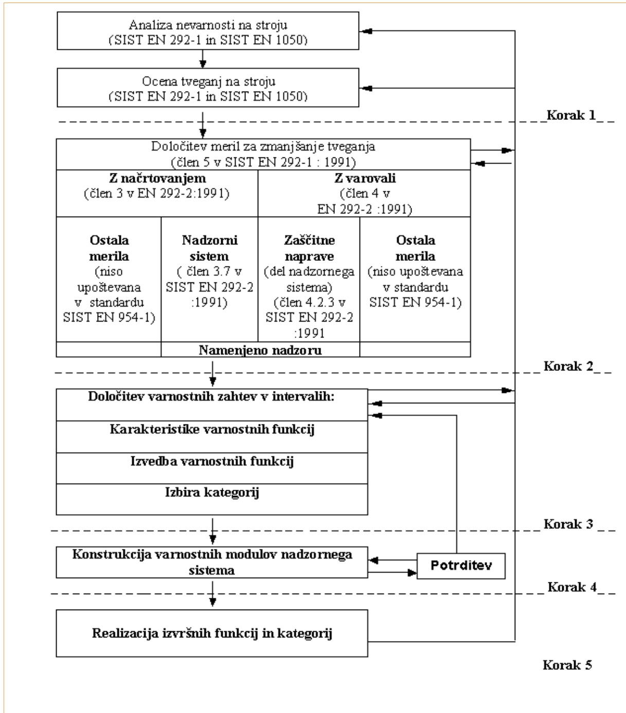
Slika 13.19: Ponavljajoč proces konstruiranja varnostnih modulov nadzornega sistema
