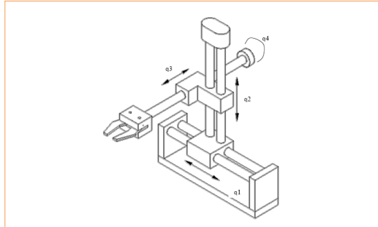
Slika 6.1: Konstrukcija kartezičnega robota
