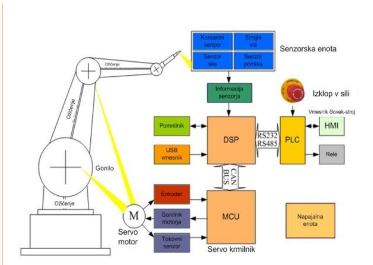
Slika 5.1: Zgradba robotskega sistema
