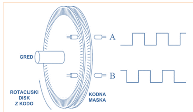
Slika 8.15: Disk z resicami in izhodni električni signali
