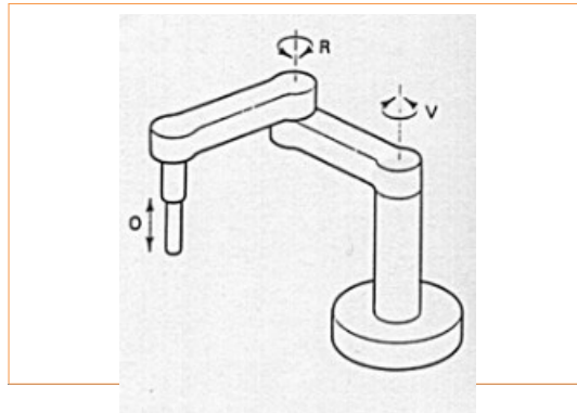
Slika 6.13: Konstrukcija scara robota
