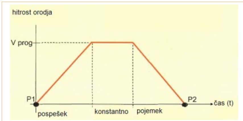
Slika 10.10: Trapezni profil hitrosti pri CIRC-gibu robota
