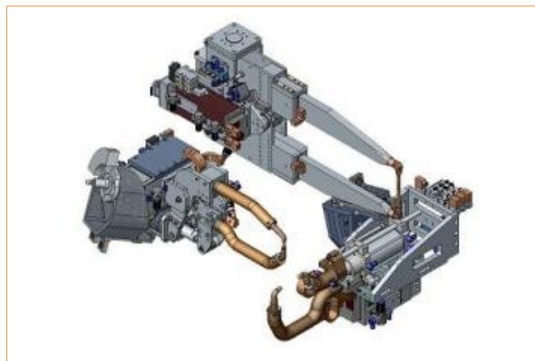
Slika 7.3: Kleščna in c-varilna varilna pištola
