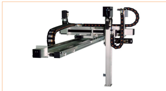
Slika 6.3: Primer kartezičnega robota
