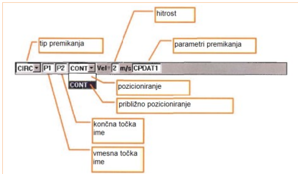
Slika 10.11: Programiranje CIRC-giba
