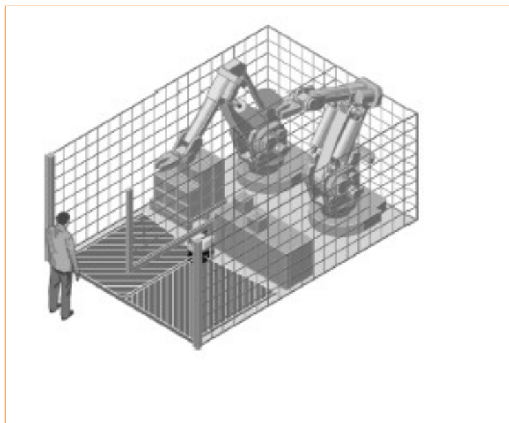
Slika 13.11: Varovanje dveh neodvisnih robotskih celic
