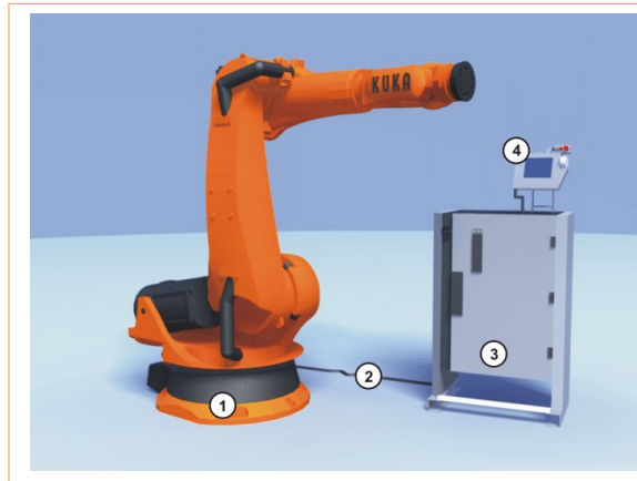
Slika 17.1: Robotsko krmilje
