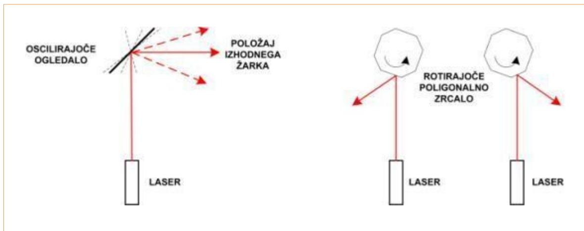
Slika 13.5: Oscilirajoče zrcalo in rotirajoče poligonalno zrcalo
