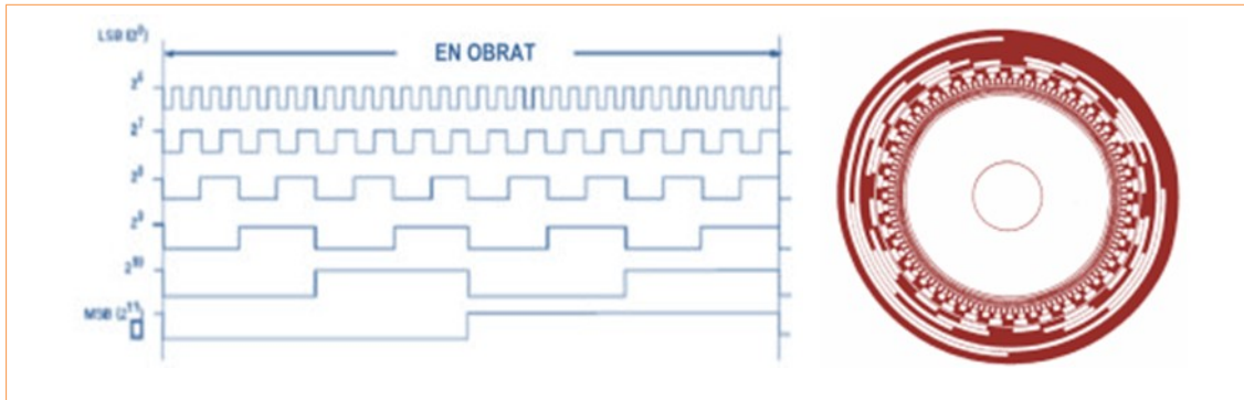
Slika 8.19: Kodiranje z binarno kodo
