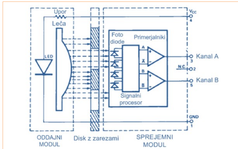
Slika 8.14 : Principalna zgradba optičnega inkrementalnega dajalnika stanja
