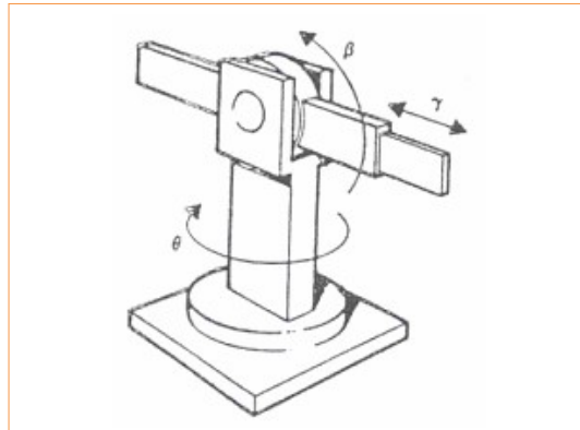
Slika 6.7: Konstrukcija sferičnega robota
