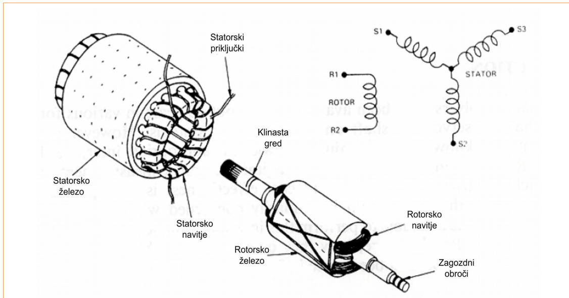
Slika 8.21: Zgradba resolverja
