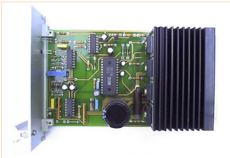
Slika 8.3: Servopogon (regulator+ojačevalnik)
