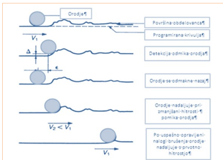
Slika 7.12: Korekcija poti ob uporabi senzorja sile ali brez njega
