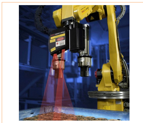
Slika 12.3: Primer robotskega strojnega vida 1
