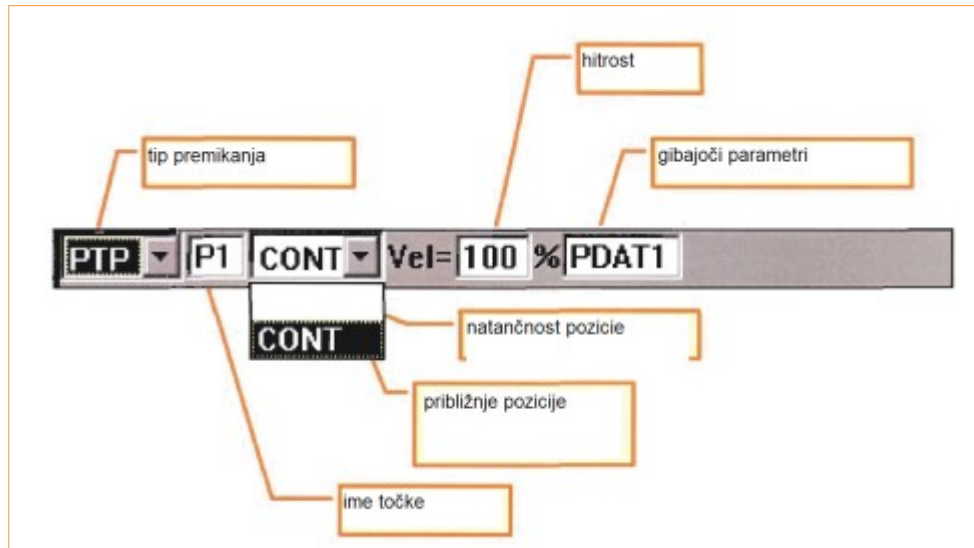
Slika 10.4: Programiranje PTP-giba
