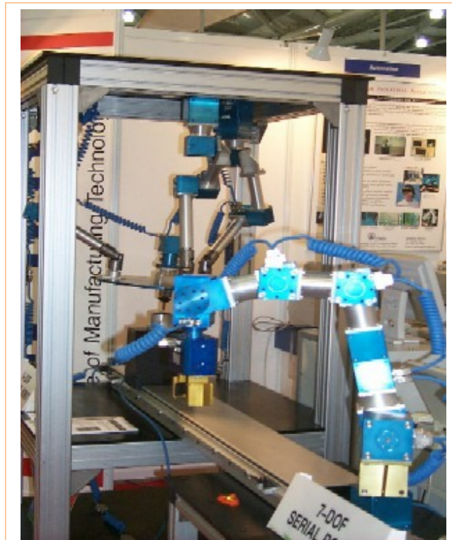
Slika 6.21: Primer modularnega robota - paralelni manipulator
