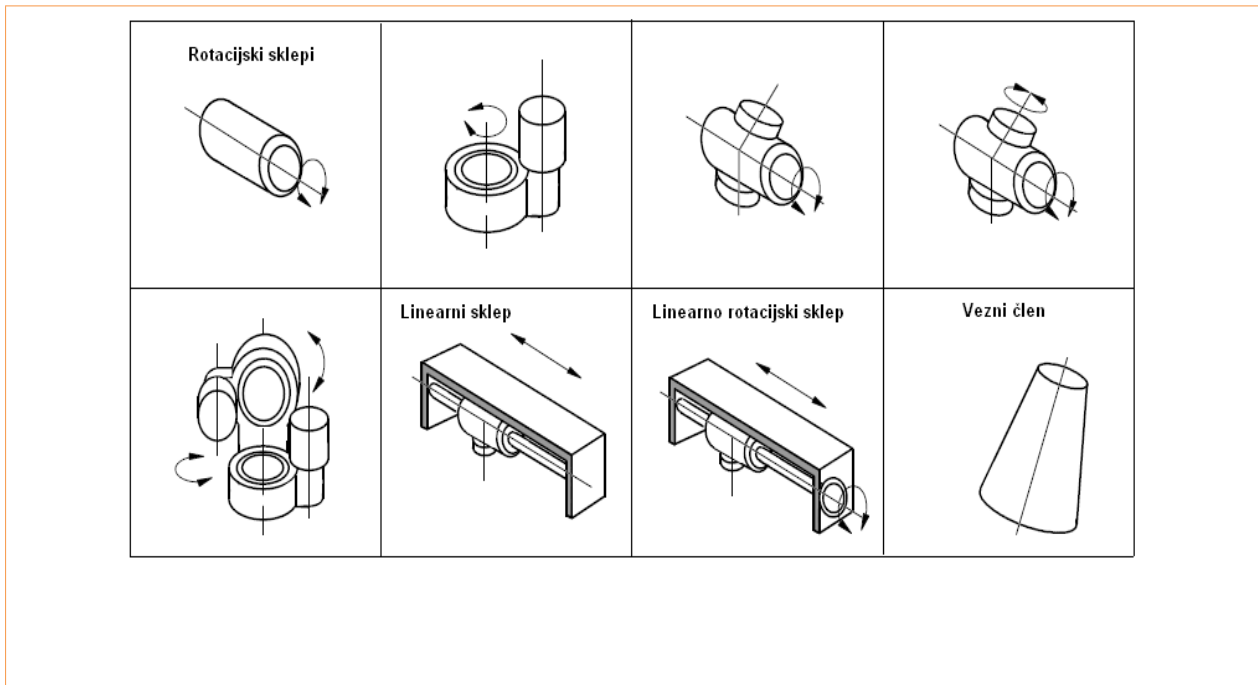
Slika 6.19: Vrste sklepov modularnih robotov
