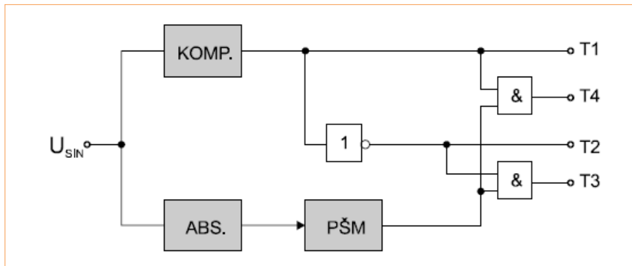
Slika 8.11: Blokovna shema PŠM
