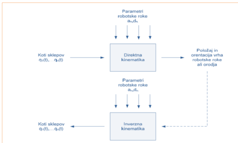
Slika 8.2: Kinematika robotske roke
