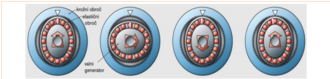
Slika 8.25: Harmonsko gonilo
