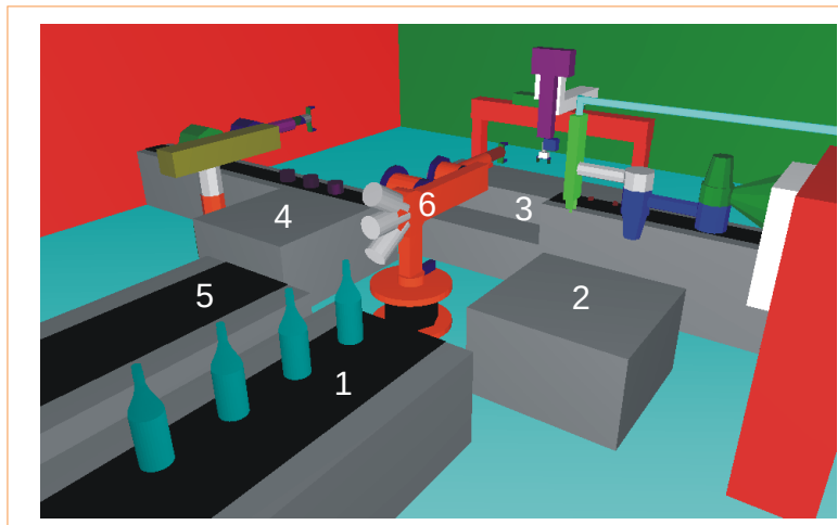
Slika 14.5: Simulacija v programu WinRobSim
