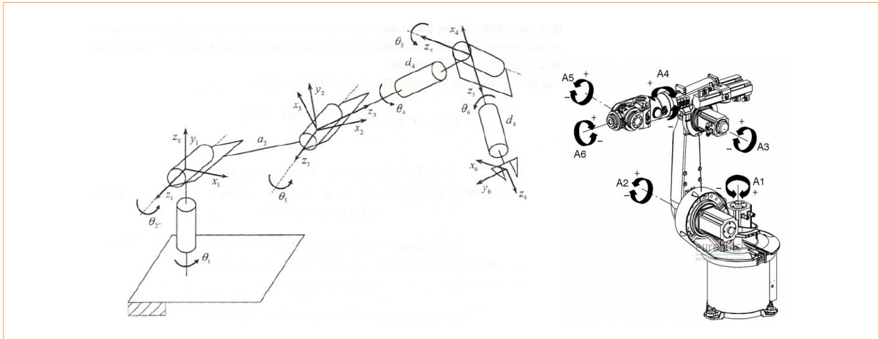
Slika 8.2: Odprta kinematična veriga robota
