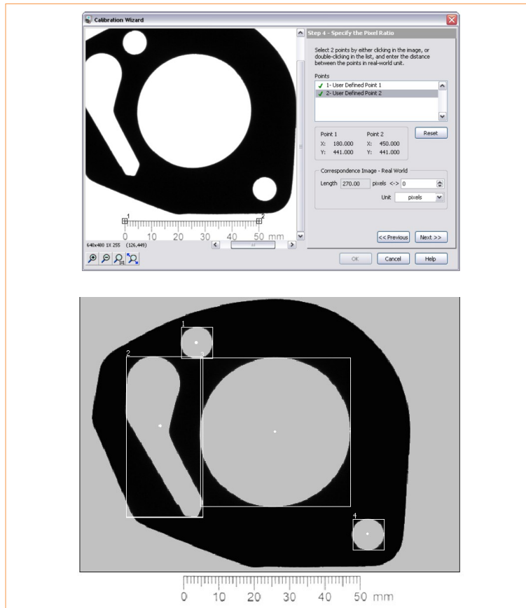
Slika 12.5: Nastavitev parametrov strojnega vida - na sliki meritev prisotnosti malih lukenj
