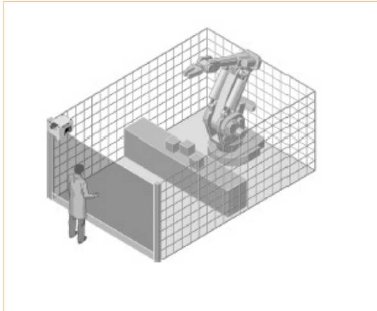
Slika 13.10: Varovanje dostopnega mesta do robota
