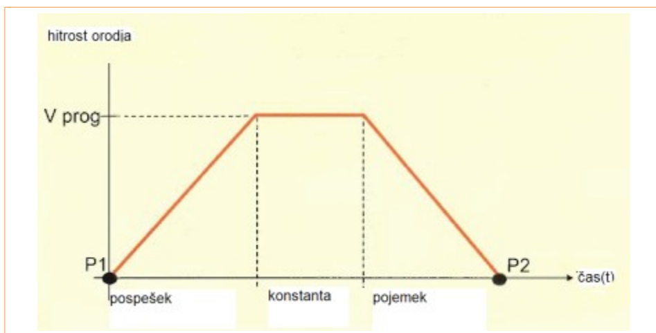
Slika 10.6: Trapezni profil hitrosti pri LIN-gibu robota
