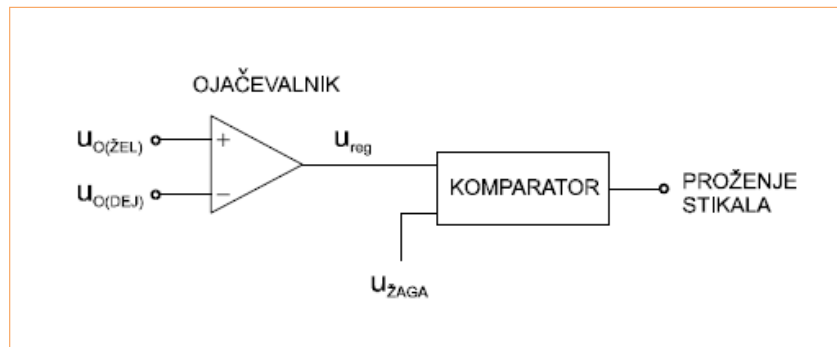
Slika 8.8: Pulznoširinski modulator (PŠM)
