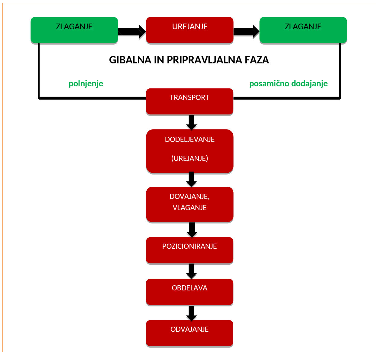
Slika 11.2: Potek izvajanja naloge prijemala
