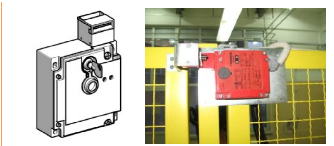
Slika 13.4: Varnostna ključavnica
