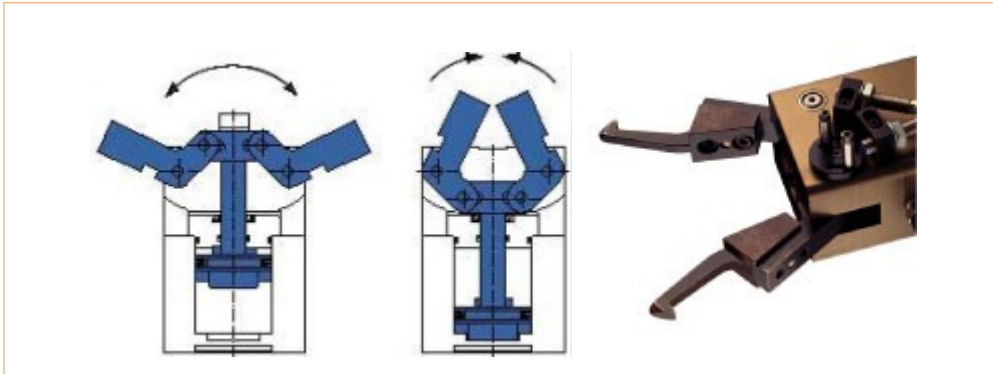
Slika 6.25: Kotna prijemala
