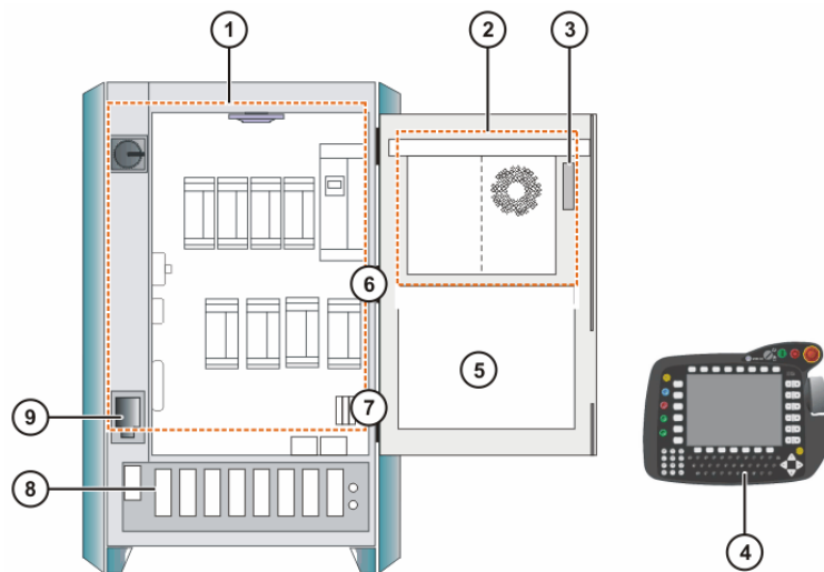
Slika 17.2: Robotski krmilnik
