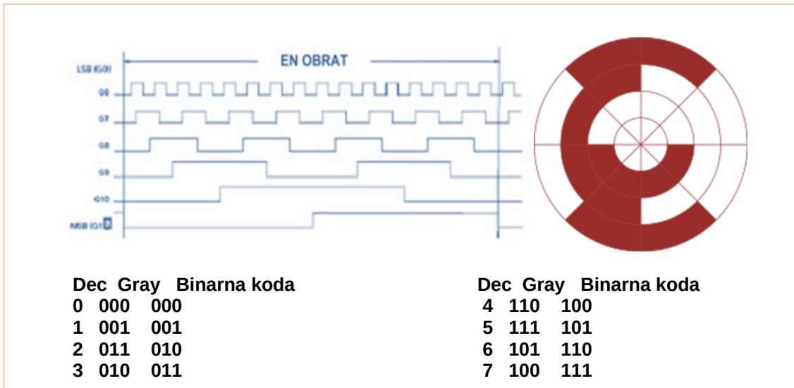
Slika 8.20: Kodiranje z Grayevo kodo
