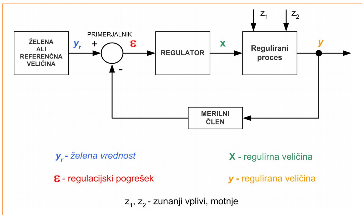
Slika 8.29: Regulacija avtomatiziranega sistema
