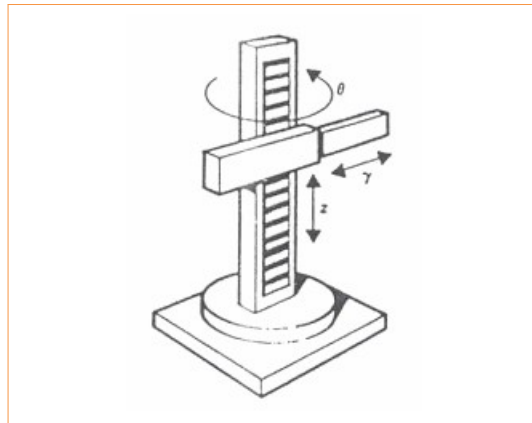
Slika 6.4: Konstrukcija cilindričnega robota
