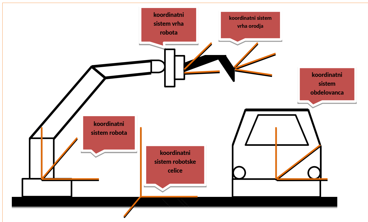
Slika 9.6: Različni koordinatni sistemi robotske celice
