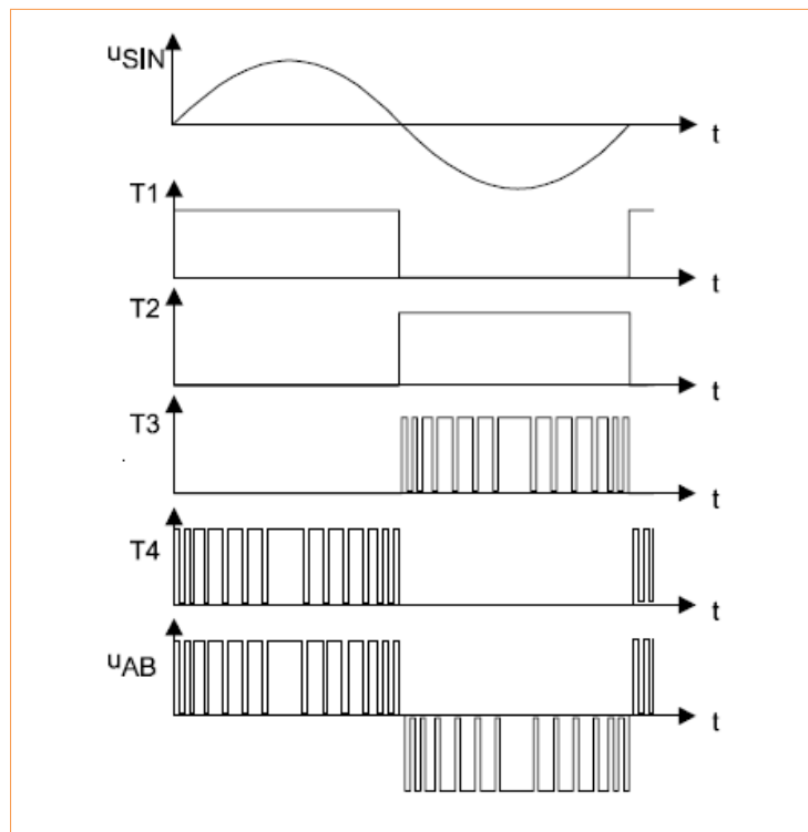
Slika 8.12: Časovni poteki proženja tranzistorjev v enofaznem tranzistorsem razsmerniku
