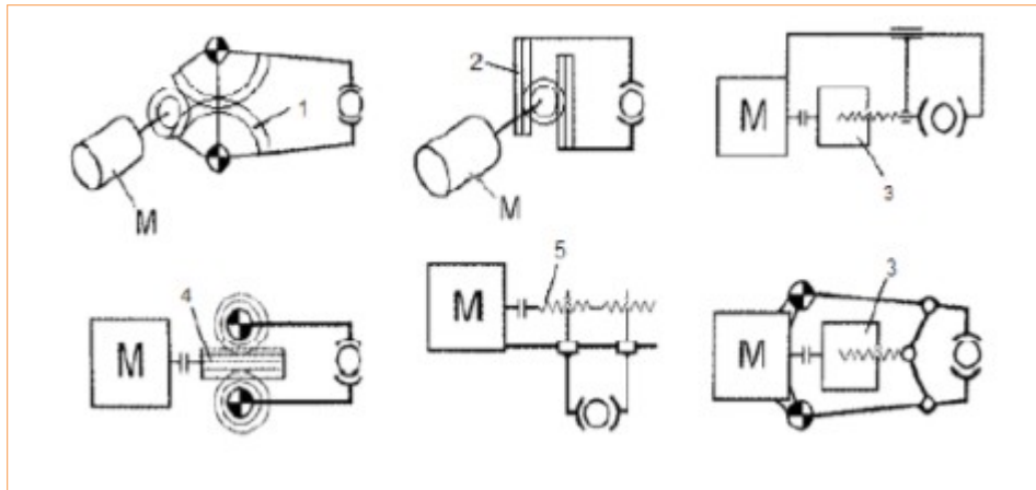
Slika 6.23: Različne izvedbe prijemal z elektromehanskim pogonom
