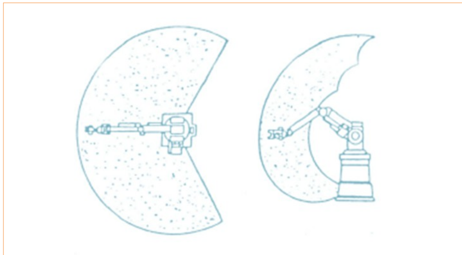
Slika 9.7: Tloris in stranski pogled delovnega prostora
