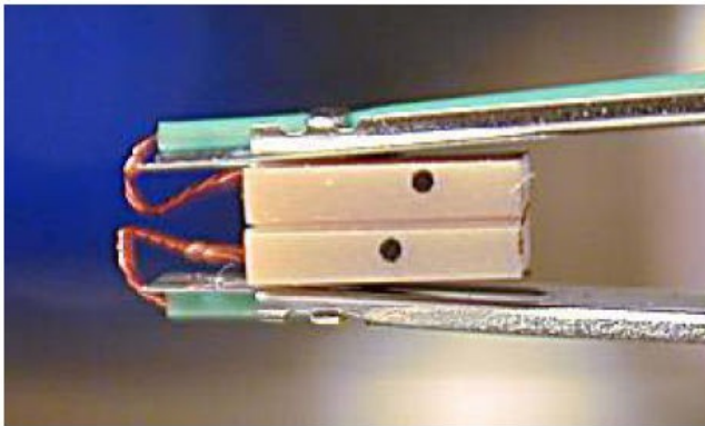
Slika 1: Bralno pisalni glavi
