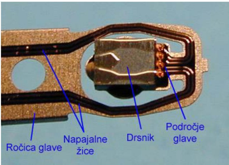
Slika 1: Zgradba bralno/pisalne glave
