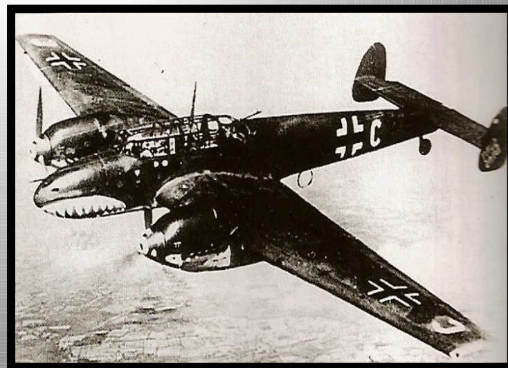
Messerschmitt ME 110C-1
